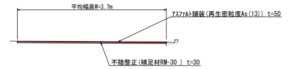
標準断面図
